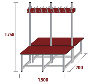
BANC-2-1500-FEN-DC COD: 79555 · 64kg · 0,6m 3 · 16 ↓
