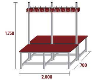
BANC-2-2000-FEN-DC COD: 79556 · 74kg · 0,62m 3 · 20 ↓
