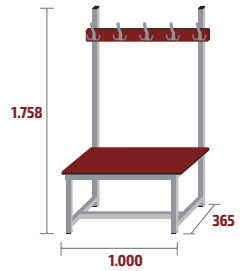
BANC-2-1000-FEN COD: 79504 · 24kg · 0,23m 3 · 5 ↓
