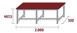
BANC-1-2000-FEN COD: 79503 · 24kg · 0,33m 3
