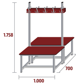
BANC-2-1000-FEN-DC COD: 79554 · 48kg · 0,46m 3 · 10 ↓
