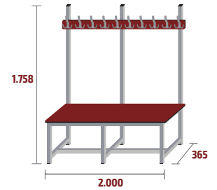
BANC-2-2000-FEN COD: 79506 · 37kg · 0,31m 3 · 10 ↓
